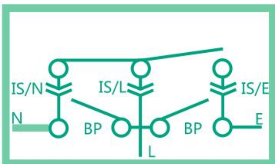
旁路隔离抽出型自动转换开关ATB
