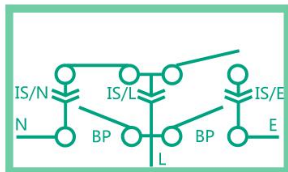
旁路隔离抽出型闭合转换开关ACTB
