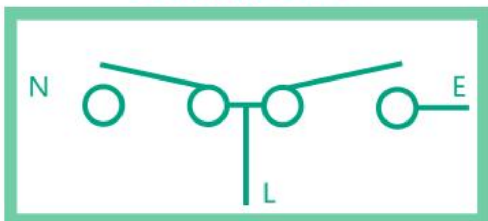
延时转换开关DTTS
