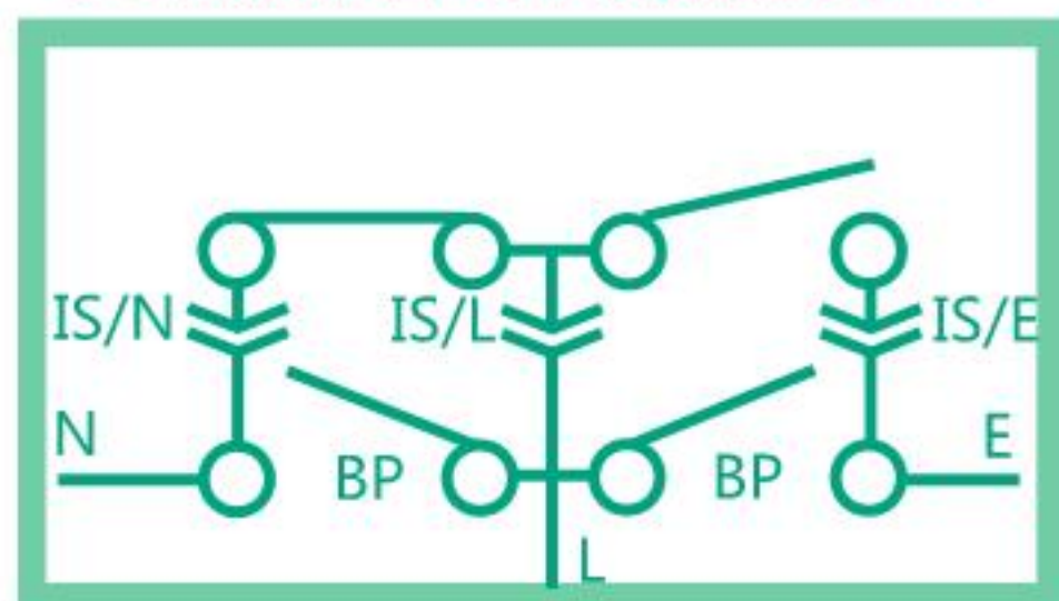
旁路隔离抽出型延时转换开关ADTB
