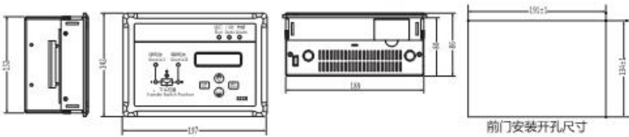
前门安装开孔尺寸
