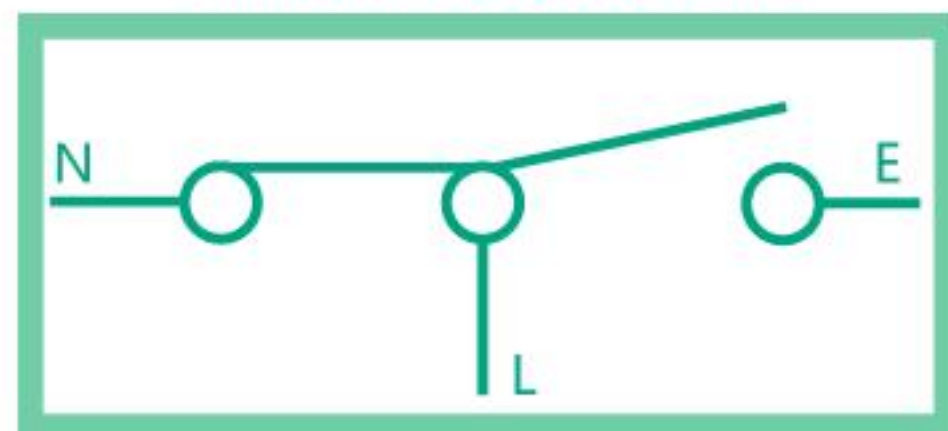
非自动转换开关NTS
